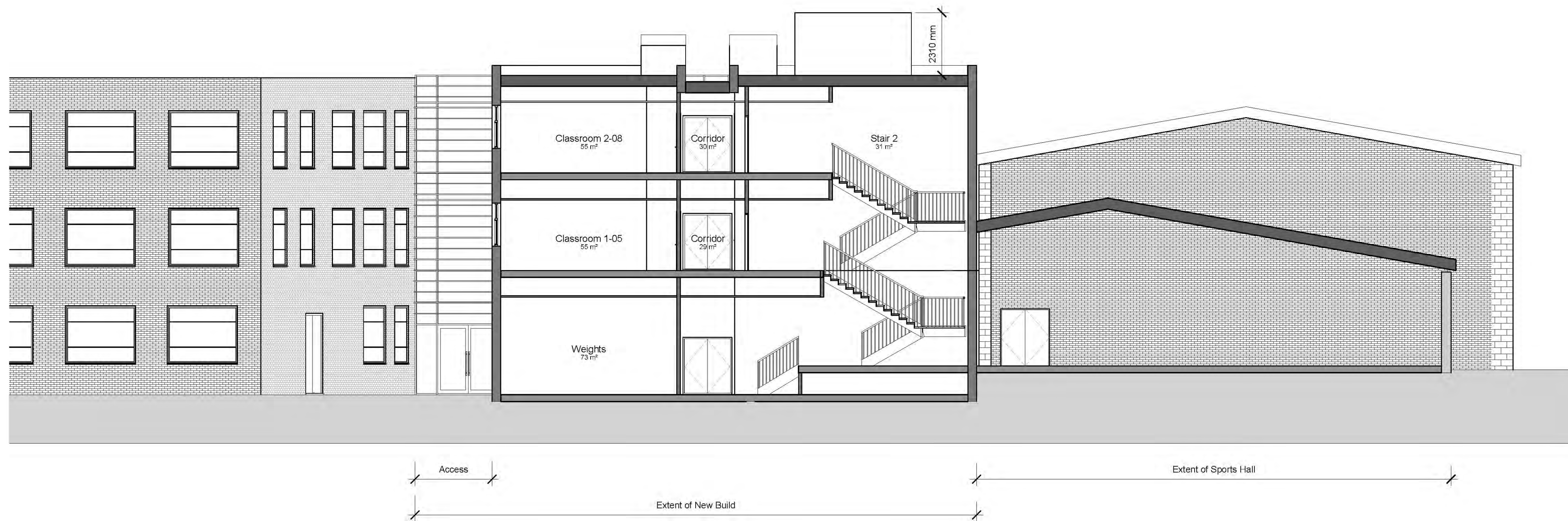
Section BB Scale - 1 : 100
